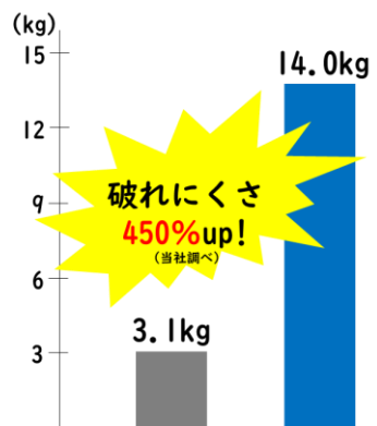
エアークラッシュ試験
